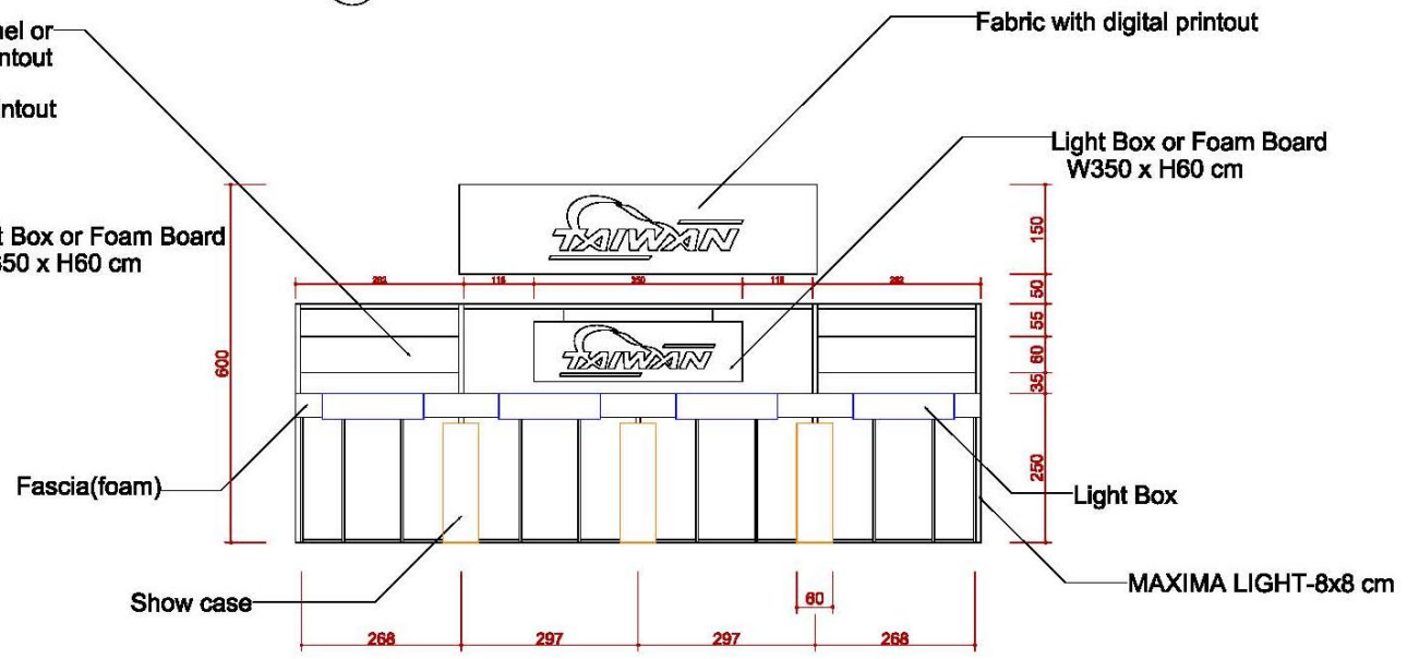
2 C-1 ELEVATION
