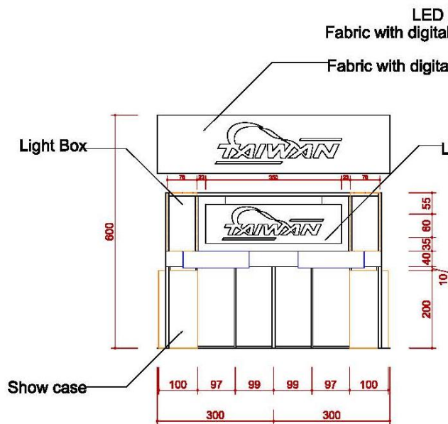
1 C-1 ELEVATION
